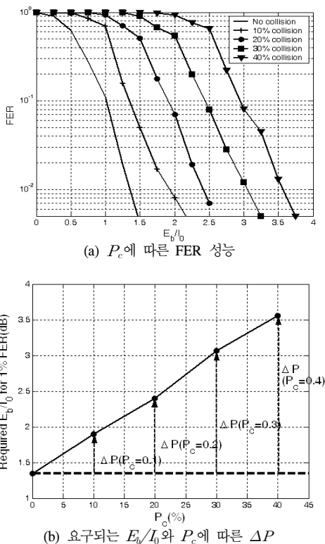
그림 5. P_c 에 따른 제안된 RFH-OFDMA 시스템의 FER 성능
