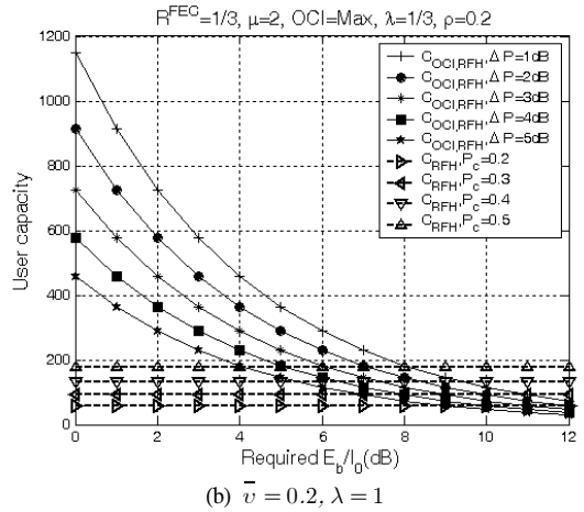
그림 4. 제안된 RFH-OFDMA 시스템의 사용자 용량
